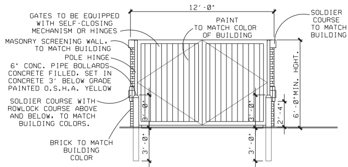
REFUSE CONTAINER ELEVATION N.T.S.
